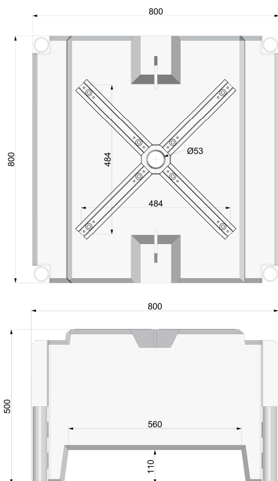
Mini Event-Block avec logements fixes pour broches
