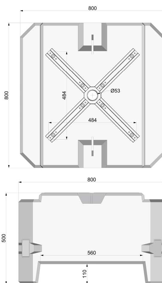
Mini Event-Block avec logements pour outrigger
